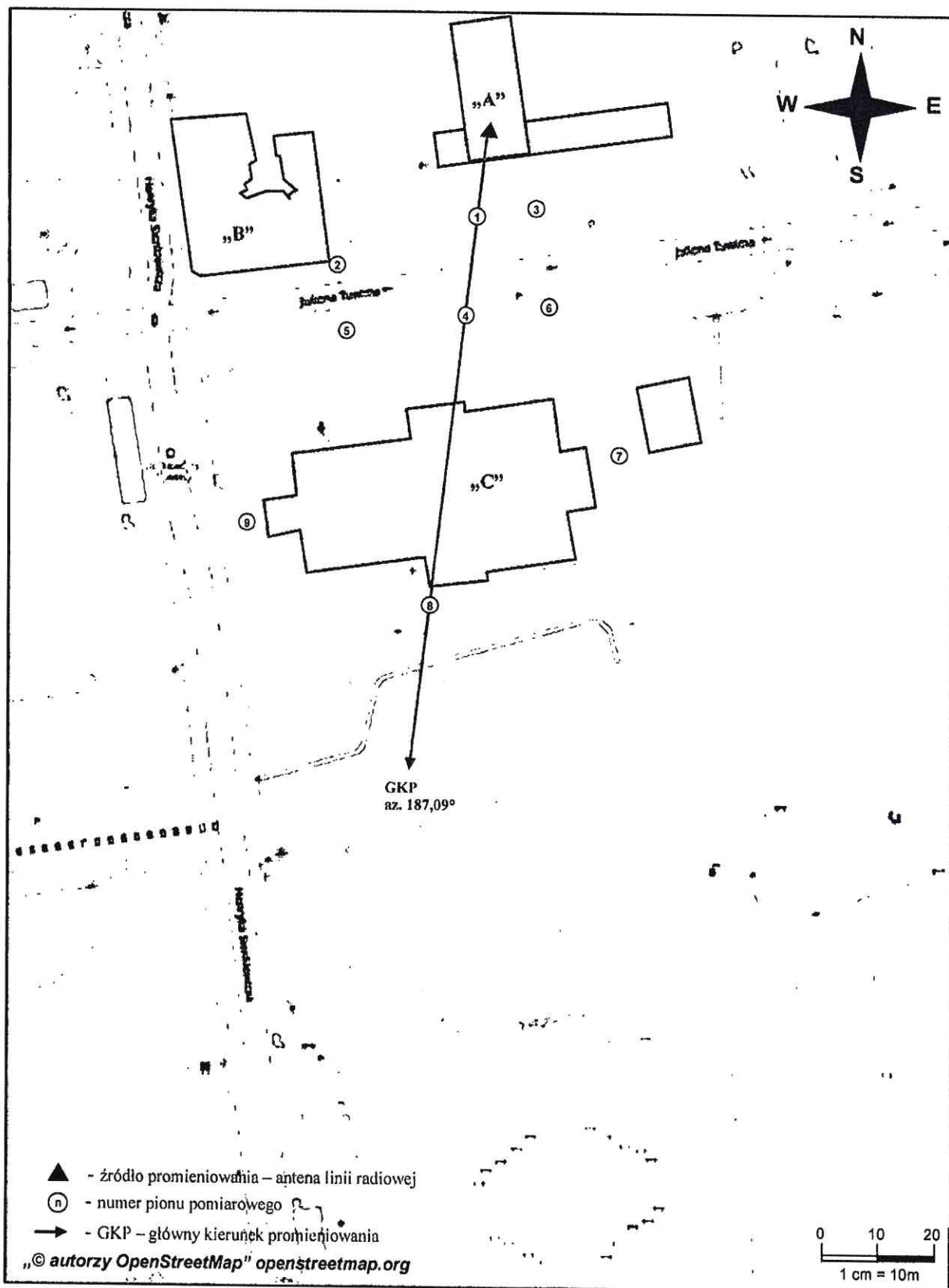
Rys. 1. Usytuowanie punktów i pionów pomiarowych w otoczeniu instalacji radiokomunikacyjnej Stacja Netia LODZB098-LODZM00077 Łódź, ul. Juliana Tuwima 22/26
