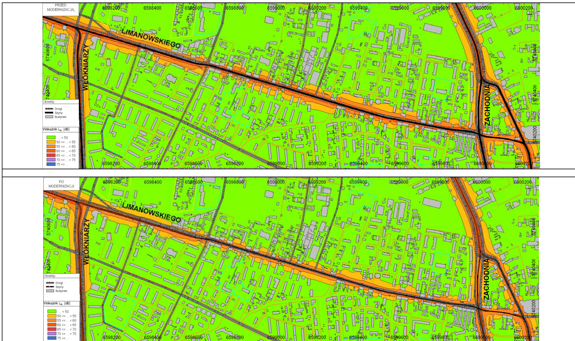
Rys. 17. Efekty modernizacji torowiska tramwajowego. Zasięg hałasu – dla wskaźnika L_N – odcinek ulicy Limanowskiego
