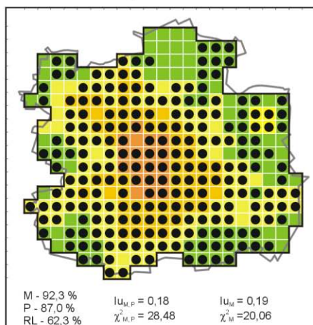
Rys. 12. Zróżnicowanie struktury przestrzennej wybranych gatunków urbanowrażliwych: a – euurbanofob, b – mezourbanofob, c – mezourbanofil, d – euurbanofil; M, P, RL – frekwencja strefach: miejskiej (iejskiej wewnętrznej i miejskiej zewnętrznej), przejściowej i rolniczo-leśnej; Iu - wskaźnik urbanobii (liczony z uwzględnieniem strefy P lub z jej pominięciem); \chi^2 - wartość testu; wg Witosławskiego 2017
