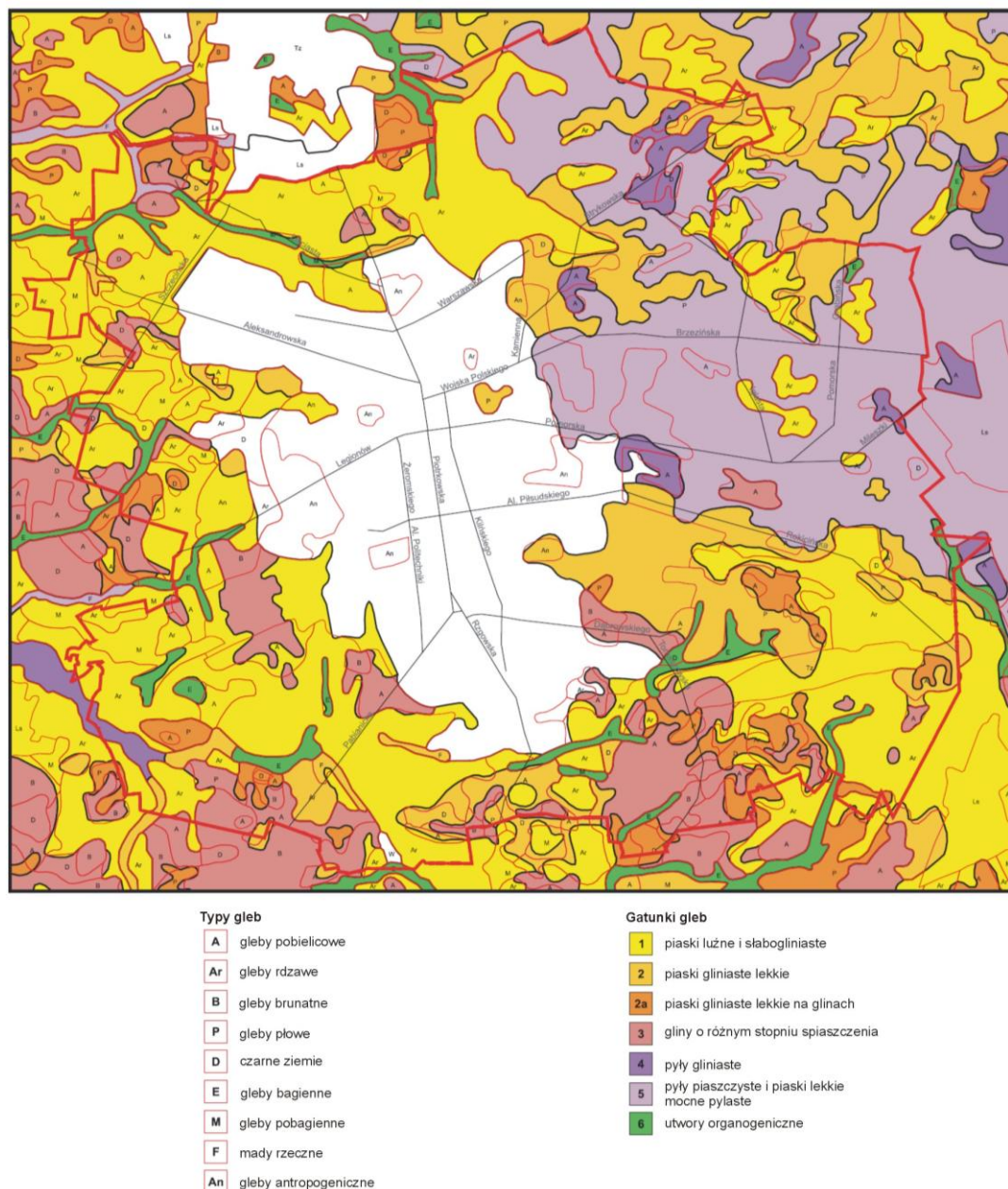
Rys. 6. Zróżnicowanie przestrzenne typów i gatunków gleb w Łodzi (wg Laskowskiego i Iwańcza 2002 zm.)
