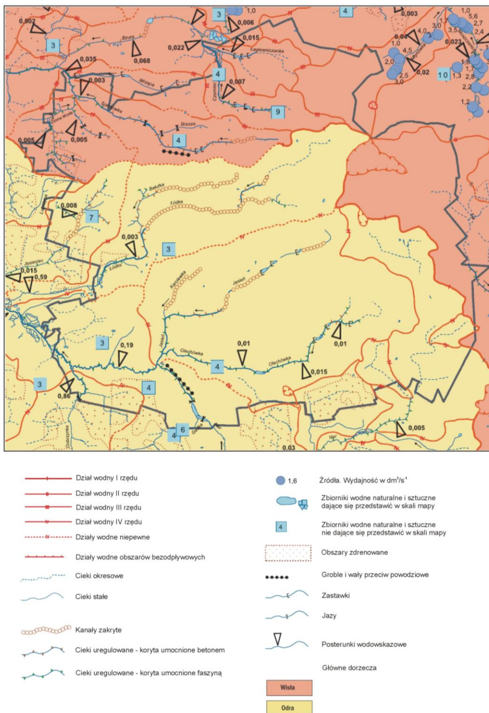
Rys. 2. Sieć rzeczna Łodzi (wg Jokiela i Maksymiuka 2002 zm.)
