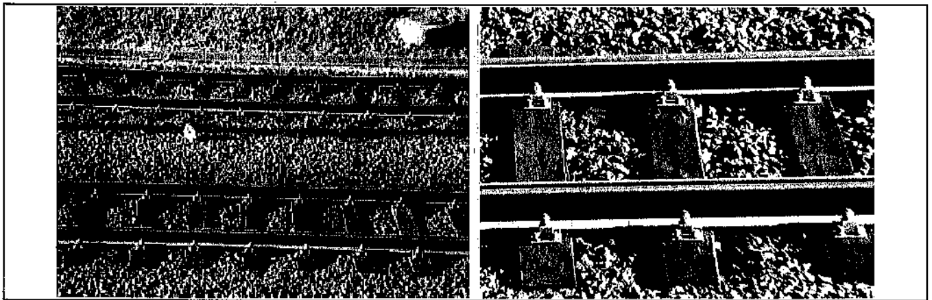
Rys. 30 Torowisko tramwajowe o sztywnym mocowaniu szyn bezстыkowych, podkładach drewnianych i podsypce (materiały własne)
