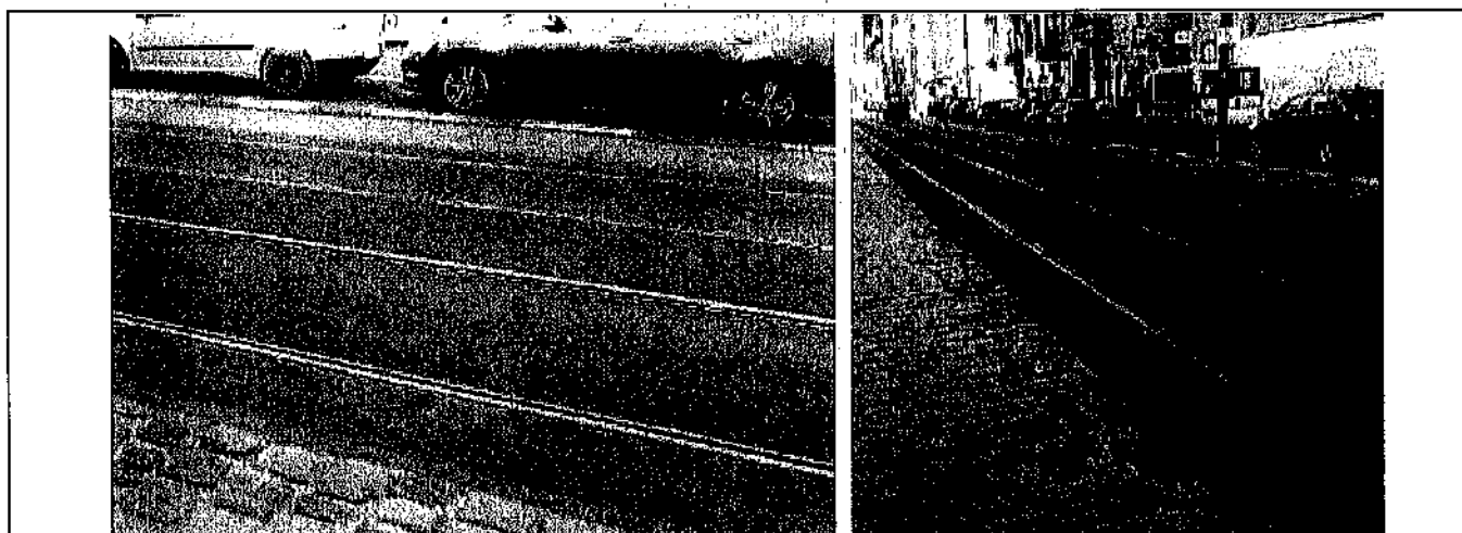
Rys. 29 Przykład zmodernizowanej drogi – częściowa wymiana nawierzchni w jezdni z kostki na asfalt wzdłuż torowiska tramwajowego umożliwia cichszy przejazd samochodem (materiały własne)
