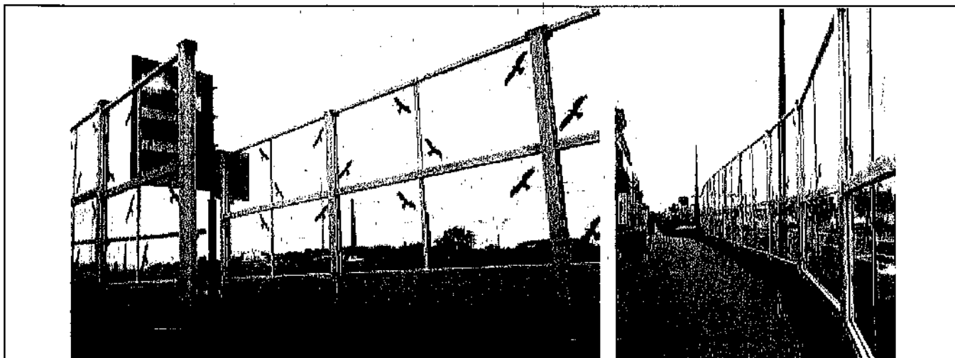
Rys. 39 Przezierne ekrany przeciwhałasowe odbijające (na zakładkę) w pobliżu zabudowy mieszkaniowej (materiały własne)
