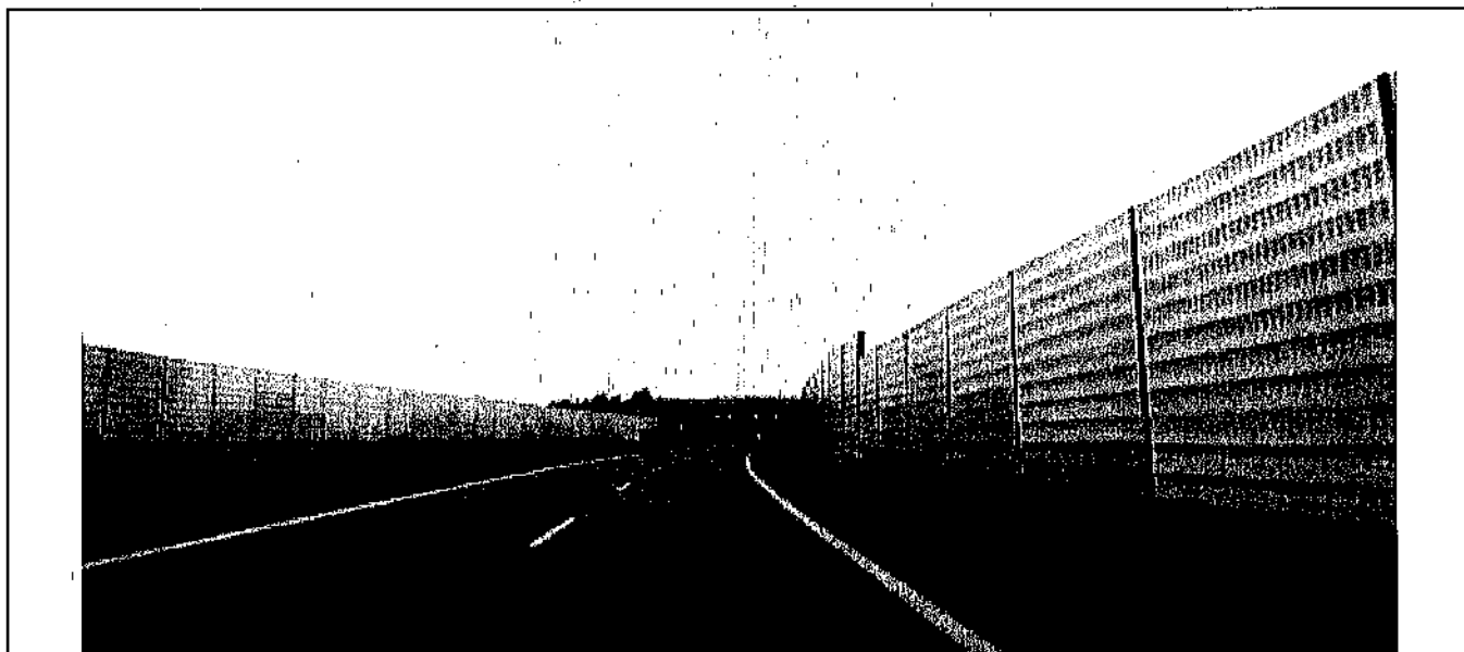
Rys. 42 Ekran przeciwhałasowe pochłaniające zbudowane z kasetonów (materiały własne)
