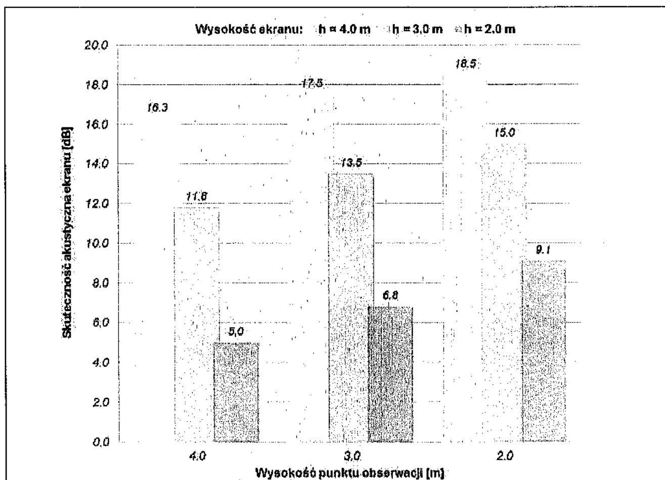
Rys. 33 Skuteczność akustyczna ekranu przy odległości źródła dźwięku od ekranu równej 4,0 m oraz punktu obserwacji od ekranu - 10,0 m (materiały własne; kolorystyka słupków zgodna z tabelą 33)
