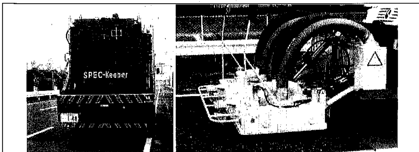
Rys. 65 Po lewej - samochód do czyszczenia cichych nawierzchni; po prawej - czyszczenie nawierzchni przy wykorzystaniu sprężonego powietrza (źródło: Noise reducing pavements in Japan - study tour report , Danish Road Institute, 2005, DRI-DWW noise abatement program)
