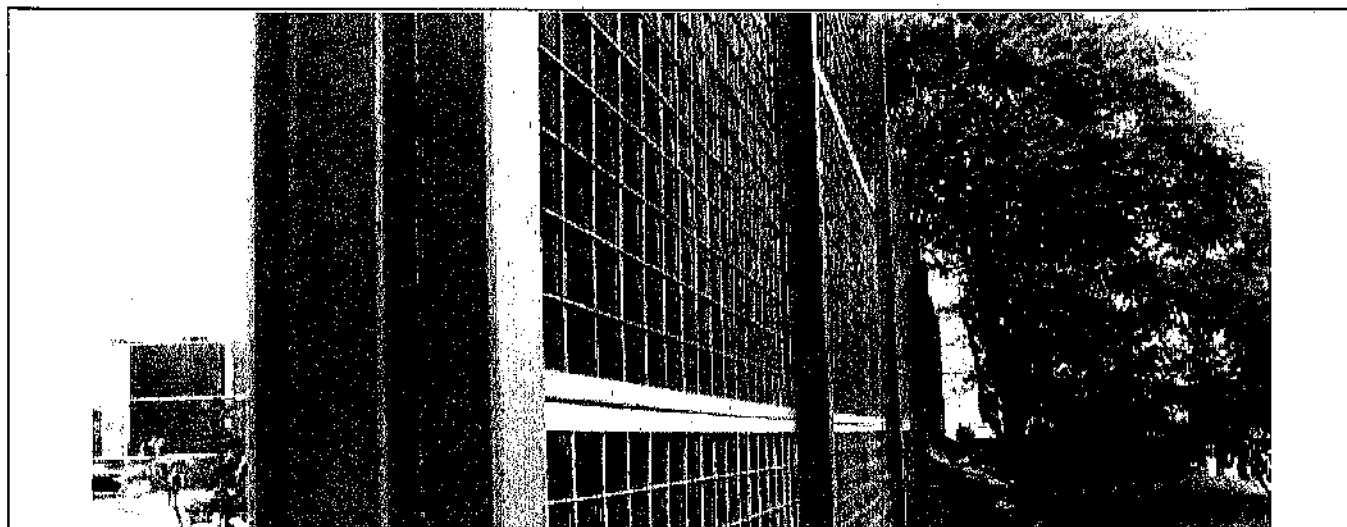
Rys. 41 Ekran przeciwhałasowy pochłaniający zbudowany z siatki z prętów stalowych oraz siatki z polietylemu, wewnątrz z wełny mineralnej i płyty drzewo-cementowej (materiały własne)
