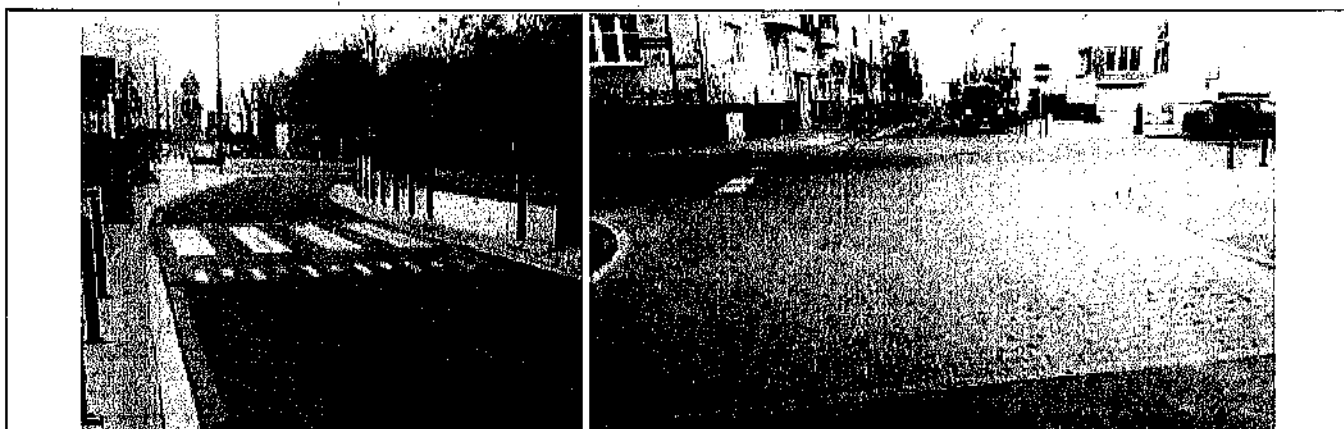
Rys. 22 Wyniesione przejście dla pieszych oraz wyniesione skrzyżowanie (materiały własne)
