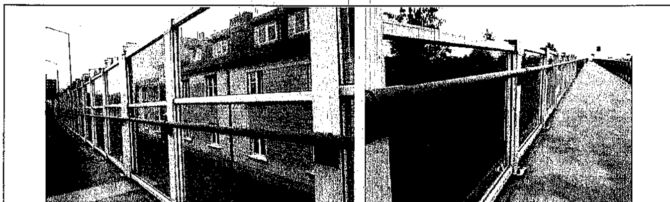
Rys. 40 Przezierny ekran przeciwhałasowy odbijający o lekkiej konstrukcji na wiadukcie (materiały własne)
