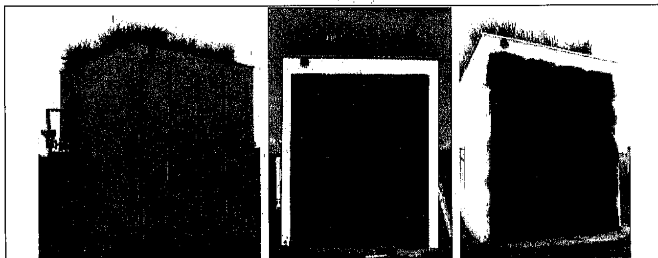
Rys. 49 Zielone ściany (green walls) o wysokim współczynniku pochłaniania jako rozwiązanie redukujące hałas w kanionach ulicznych; od lewej – Konfiguracja I – ściana z zamontowanymi słupami stalowymi, Konfiguracja II – ściana z 20 panelami ze sklejki na stalowych słupach + kieszenie z geowłókniny + podłoże; Konfiguracja III – jak w II + roślinność (źródło: jw.)
