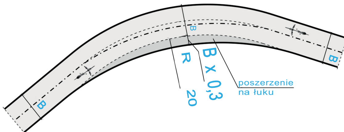
Rysunek 6 Poszerzenie drogi dla rowerów na łuku o promieniu R < 20 m
