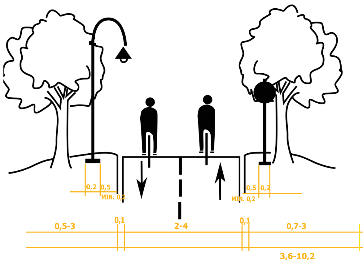
Rysunek 4 Szerokość korytarza dwukierunkowej drogi dla rowerów
