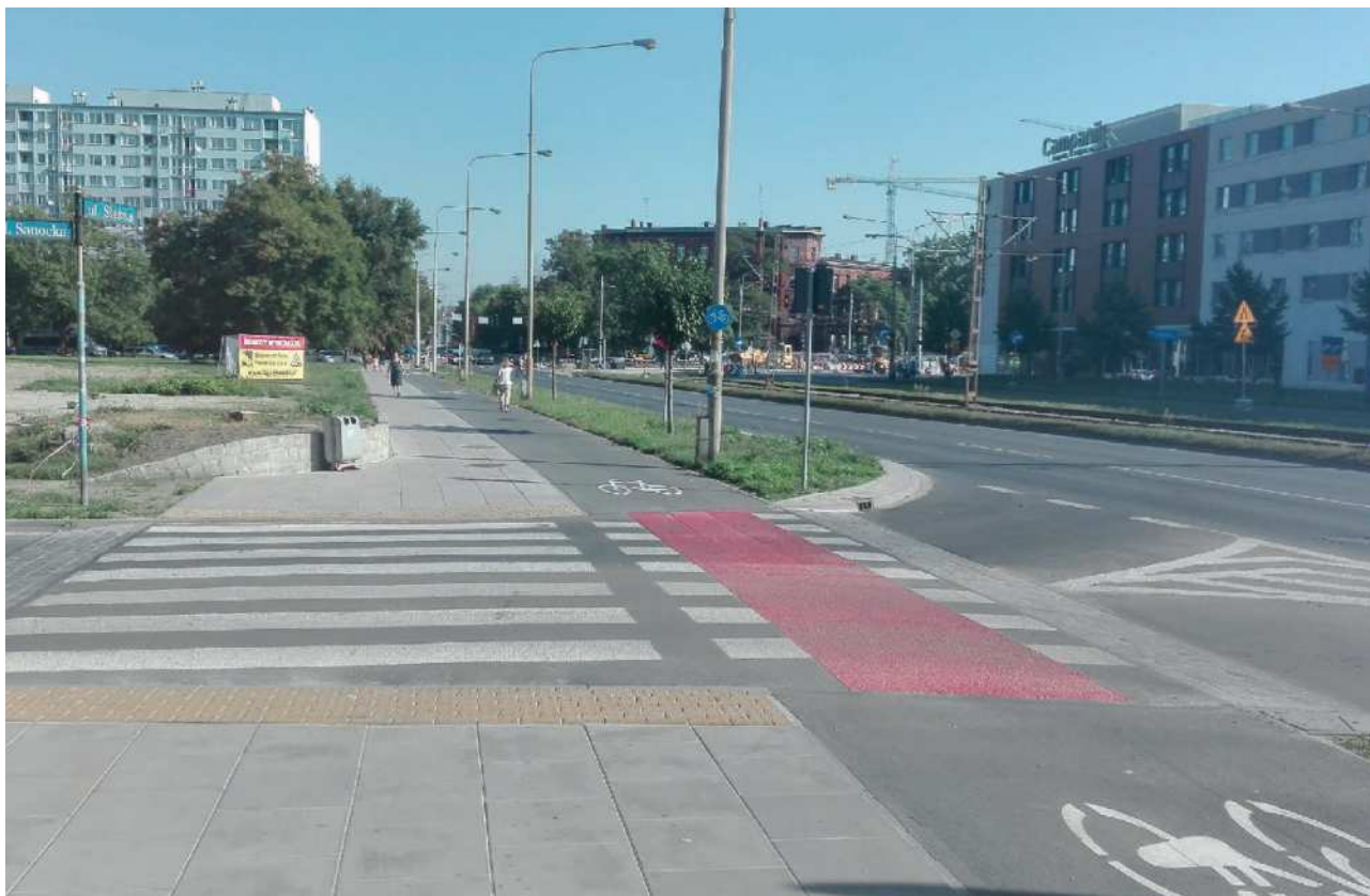
Zdjęcie 18 Ciągłość nawierzchni i niwelety drogi dla rowerów przez drogę podporządkowaną. Wrocław, Polska
