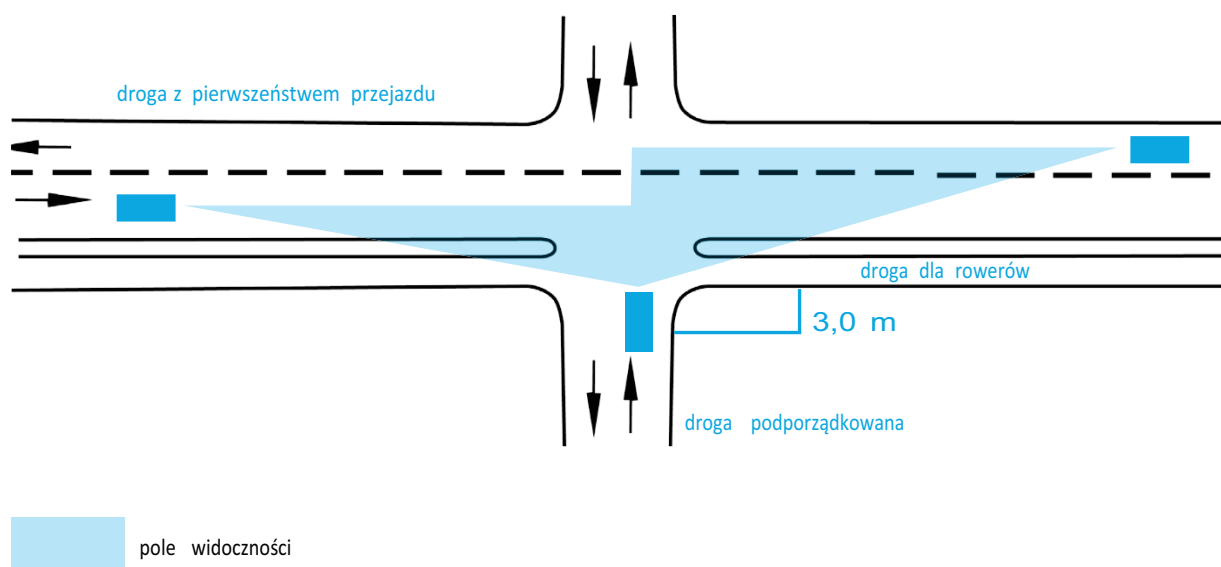
Rysunek 8 Odległość widoczności na skrzyżowaniach - droga dla rowerów wzdłuż drogi głównej
