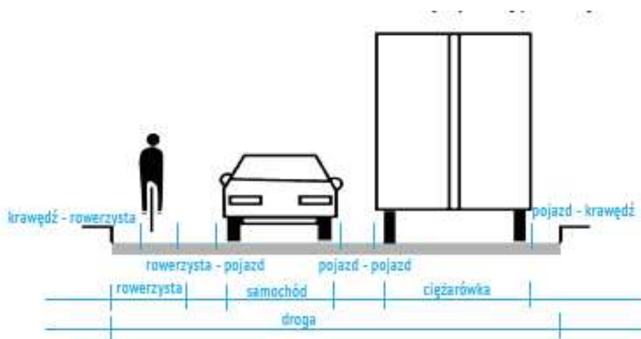
Schemat graficzny 2 Rekomendowane szerokości jezdni w strefie ruchu uspokojonego
