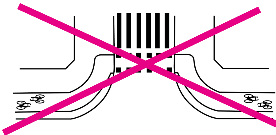
Rysunek 15 Niedopuszczalne odgięcie drogi dla rowerów przed samym przejazdem
