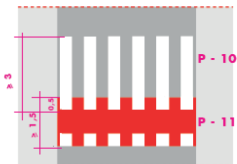
Rysunek 13 Oznakowanie przejazdu dla rowerzystów łączonego z przejściem pieszym
