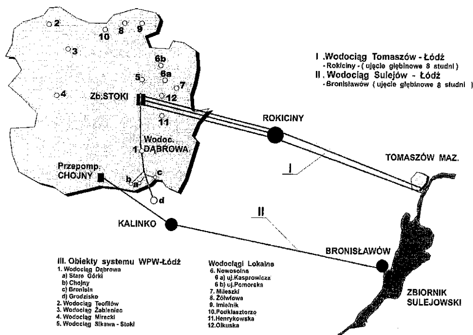
Rysunek 9 Schemat zaopatrzenia miasta Łodzi w wodę
