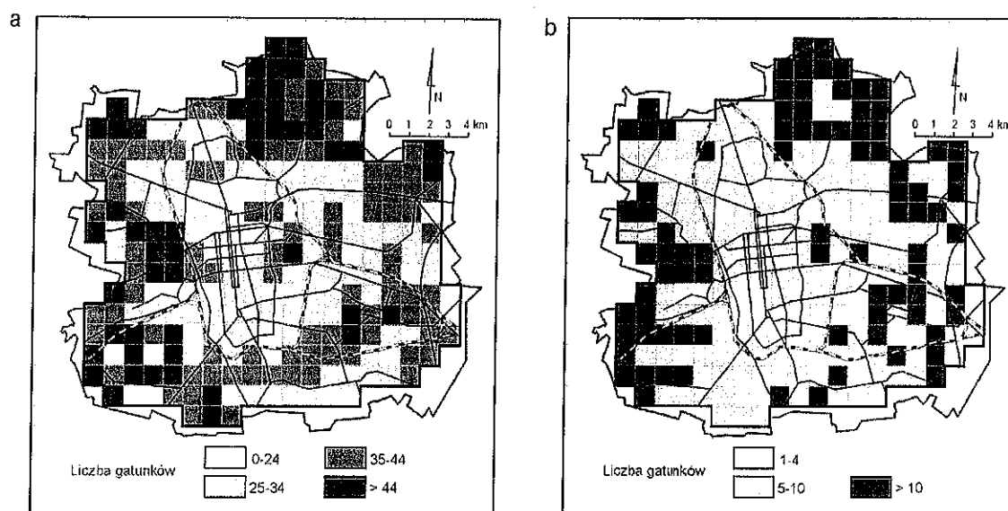
Rysunek 19 Przemianowe zróżnicowanie zagęszczenia gatunków ptaków: łęgowych (a) i kluczowych (b)
