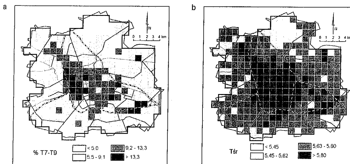
Rysunek 15 Przestrzenne zróżnicowanie udziału we florze gatunków termofilnych (a) oraz średnich wartości wskaźników temperatury (b)
