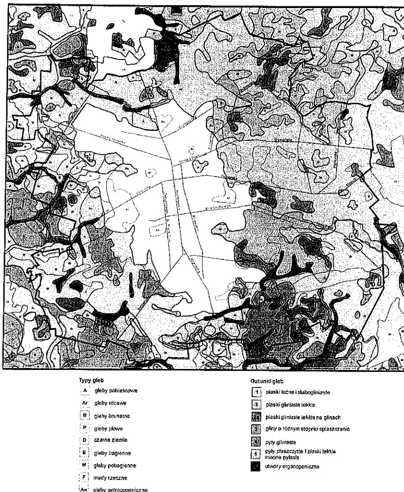
Rysunek 12 Zróżnicowanie przestrzenne typów i gatunków gleb w Łodzi
