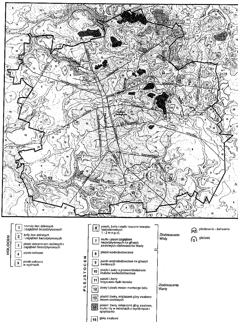
Rysunek 10 Geologiczne utwory powierzchniowe
