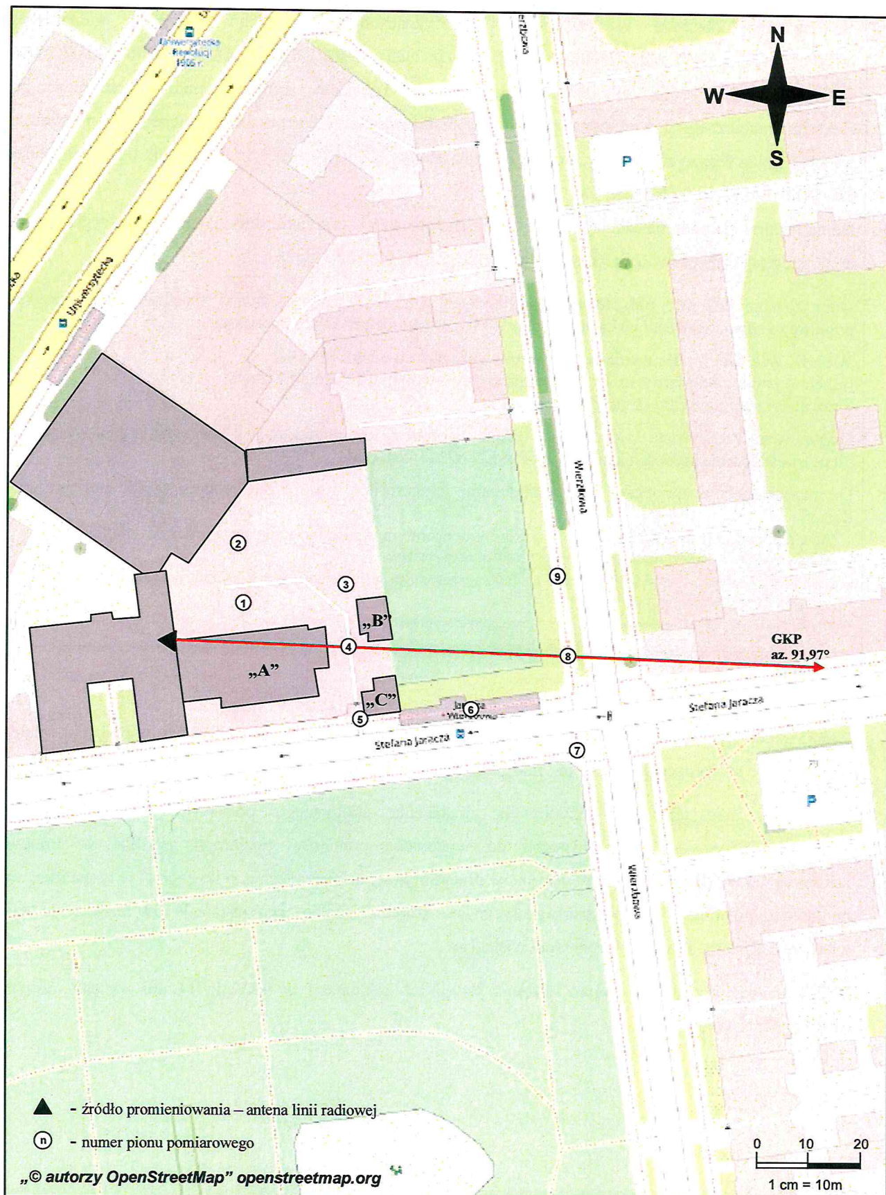
Rys. 1. Usytuowanie punktów i pionów pomiarowych w otoczeniu instalacji radiokomunikacyjnej Stacja Netia LODZD627-LODZM00476 Łódź, ul. Stefana Jaracza 82
