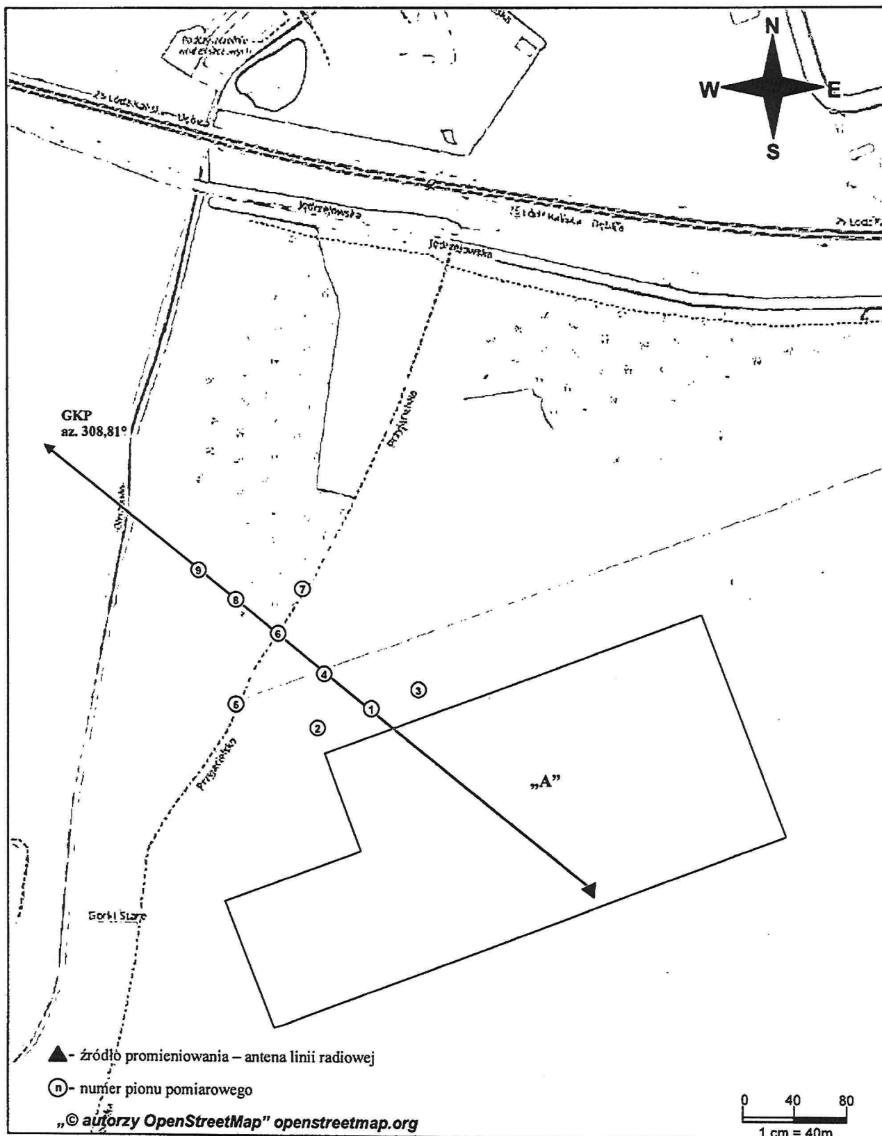
Rys. 1. Usytuowanie punktów i pionów pomiarowych w otoczeniu instalacji radiokomunikacyjnej Stacja Netia LODZD577-LODZM00470 Łódź, ul. Jędrzejowska 43
