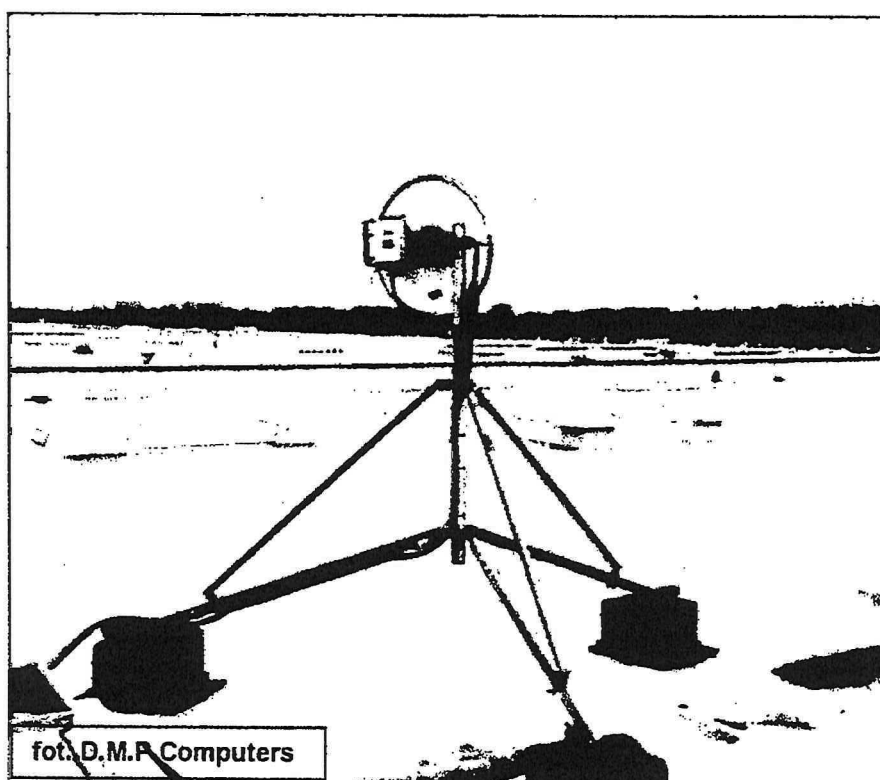
Widok instalacji radiokomunikacyjnej Stacja Netia LODZD577 - LODZM00470 Łódź, ul. Jędrzejowska 43.
