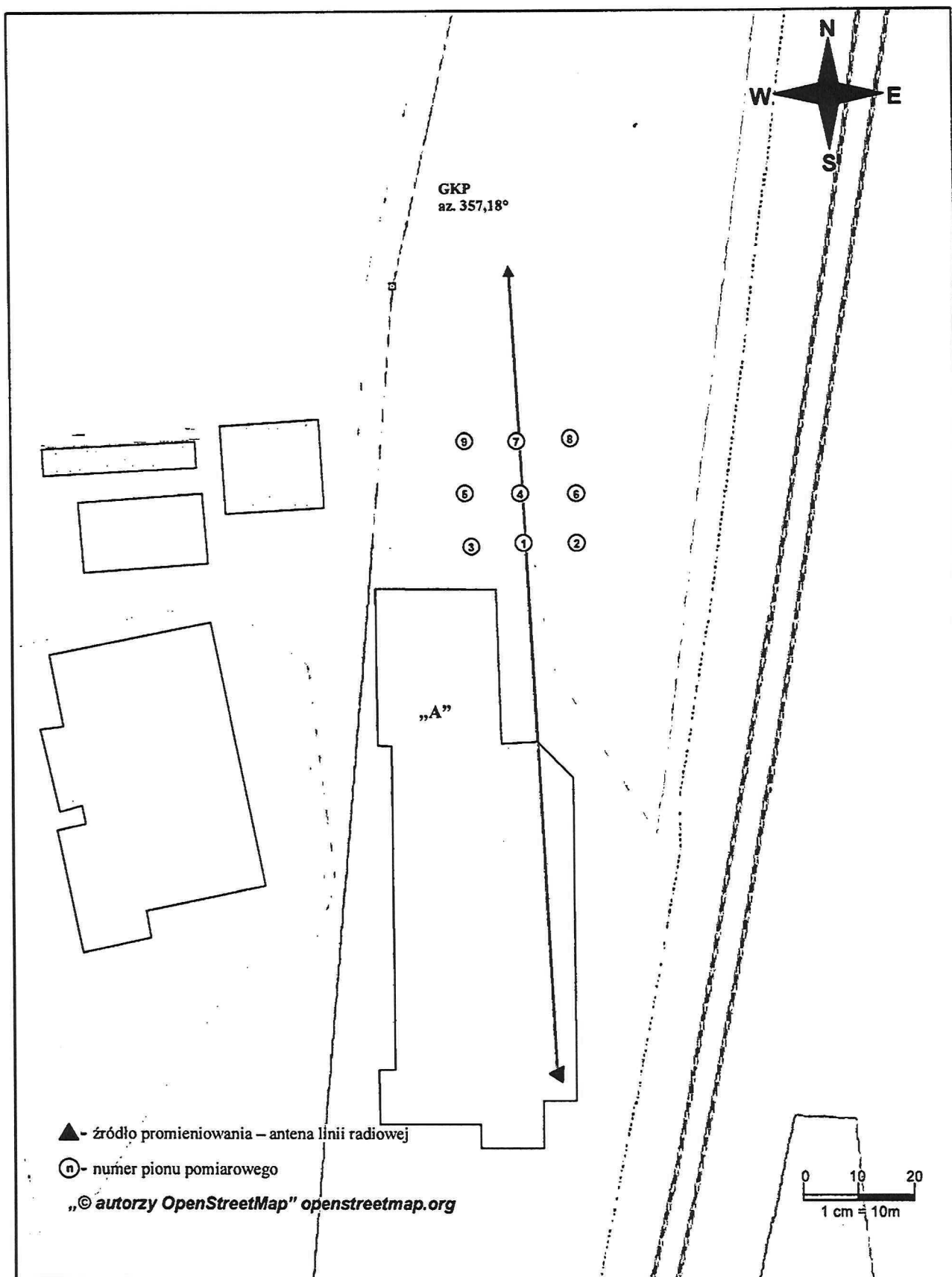
Rys. 1. Usytuowanie punktów i pionów pomiarowych w otoczeniu instalacji radiokomunikacyjnej Stacja Netia LODZD583-LODZM00471 Łódź, ul. Śląska 126D
