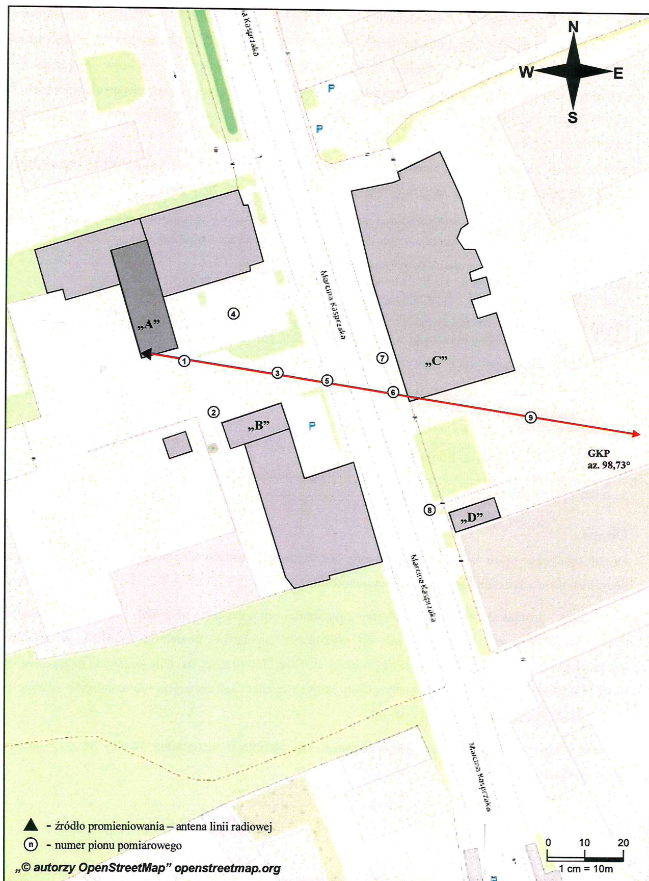
Rys. 1. Usytuowanie punktów i pionów pomiarowych w otoczeniu instalacji radiokomunikacyjnej Stacja Netia LODZD883-LODZM00488 Łódź, ul. Marcina Kasprzaka 6
