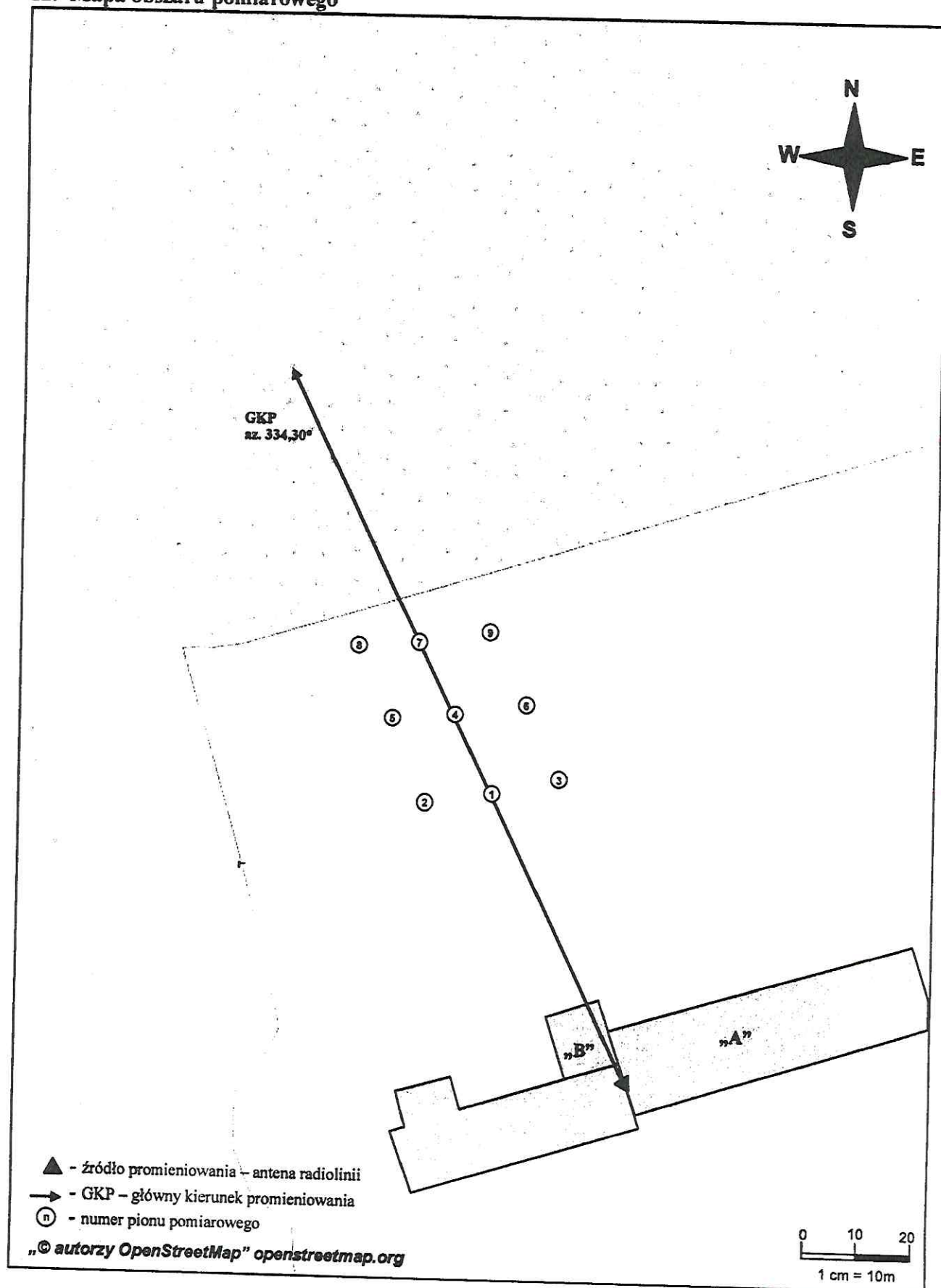
Rys. 1. Usytuowanie punktów i pionów pomiarowych w otoczeniu instalacji radiokomunikacyjnej Stacja Netia LODZD961-LODZM00494 Łódź, ul. Tomaszowska 60
