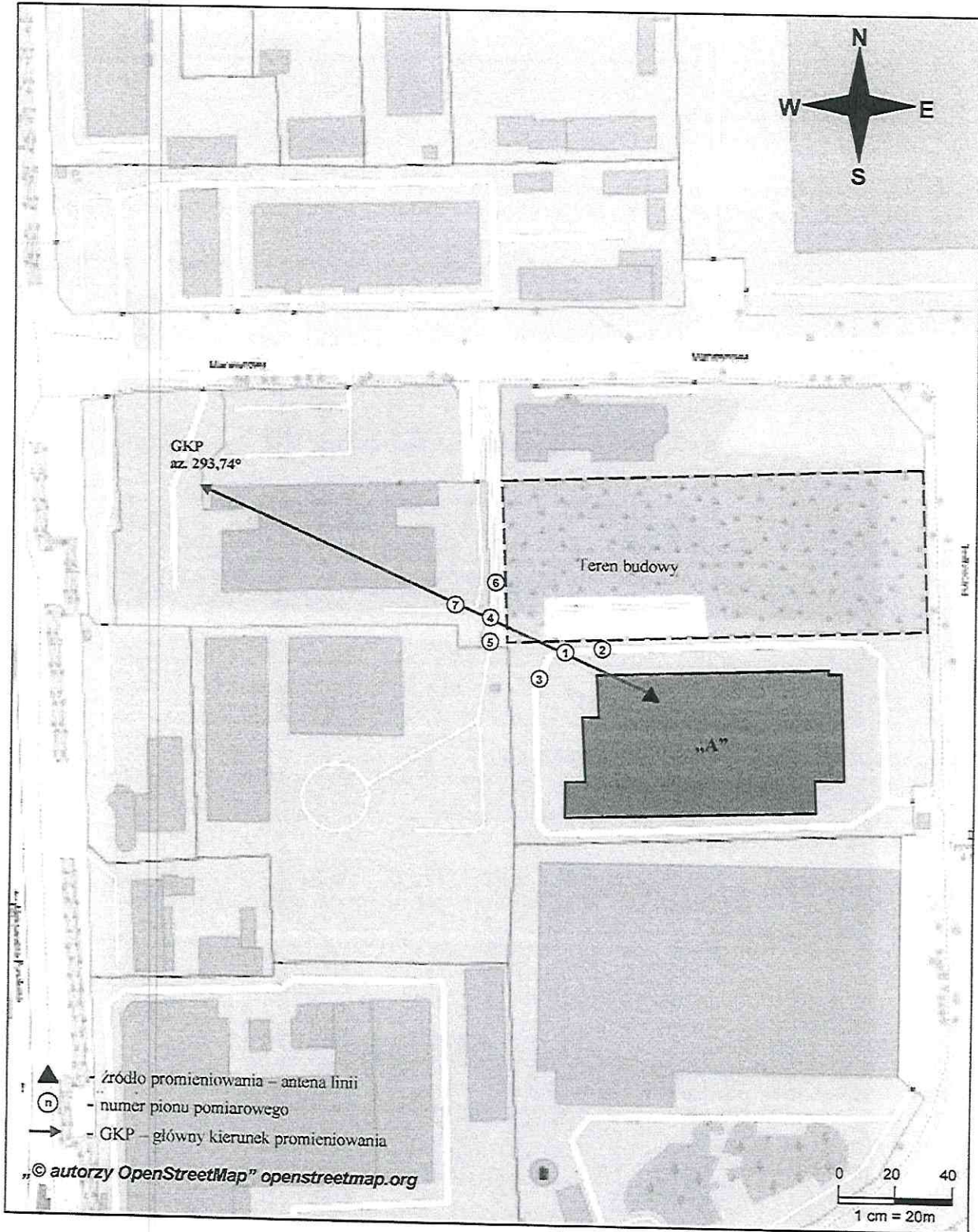
Rys. 1. Usytuowanie punktów i pionów pomiarowych w otoczeniu instalacji radiokomunikacyjnej Stacja Netia LODZB303-LODZM00284 Łódź, ul. Techniczna 5
