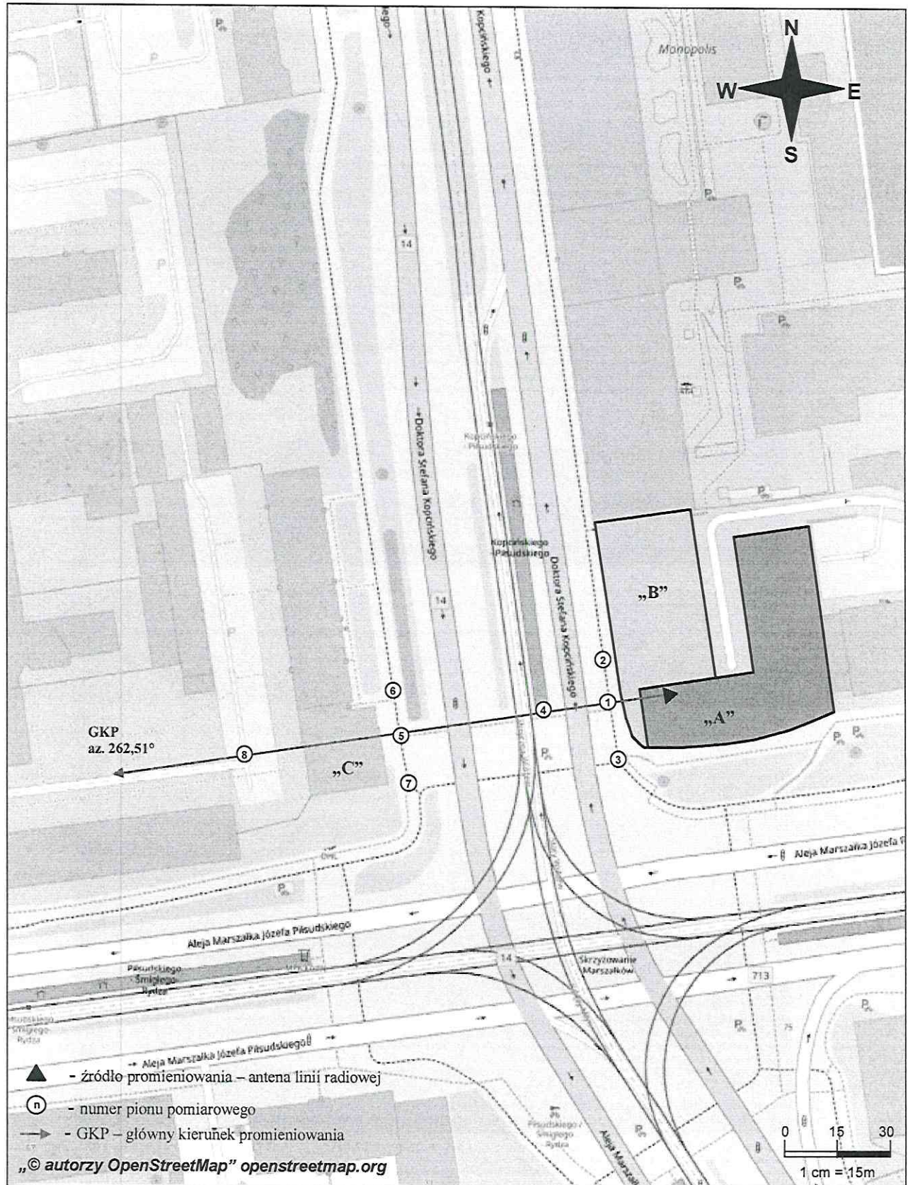
Rys. 1. Usytuowanie punktów i pionów pomiarowych w otoczeniu instalacji radiokomunikacyjnej Stacja Netia LODZB928-LODZM00501 Łódź, Aleja Marszałka Józefa Piłsudskiego 76
