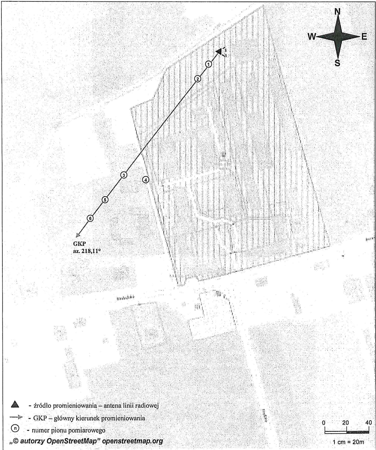
Rys. 1. Usytuowanie punktów i pionów pomiarowych w otoczeniu instalacji radiokomunikacyjnej Stacja Netia LODZB927-LODZM00444 Łódź, ul. Beskidzka 54A
